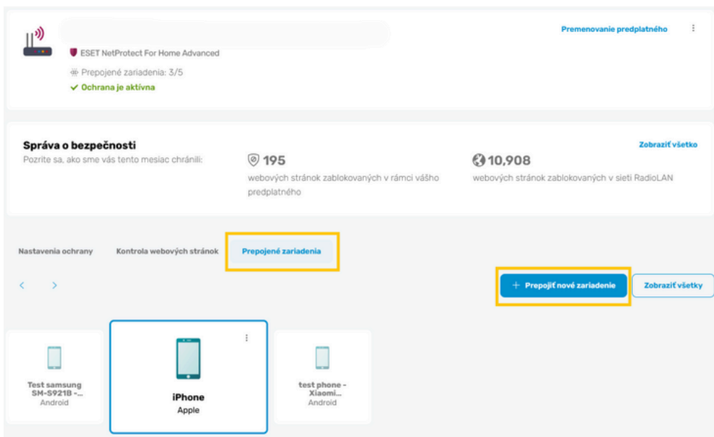
Obrázok 3 Pridanie zariadenia
