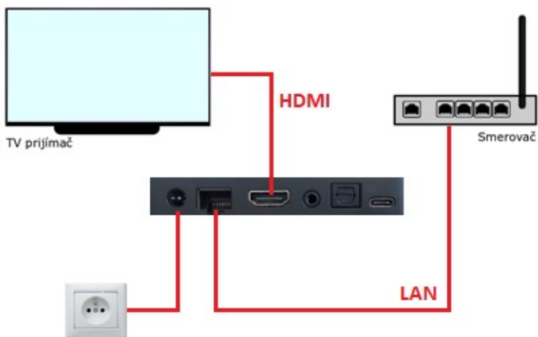
Obrázok 1 Schéma zapojenia Media boxu
